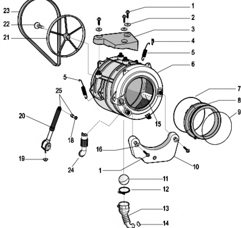
VUE B
